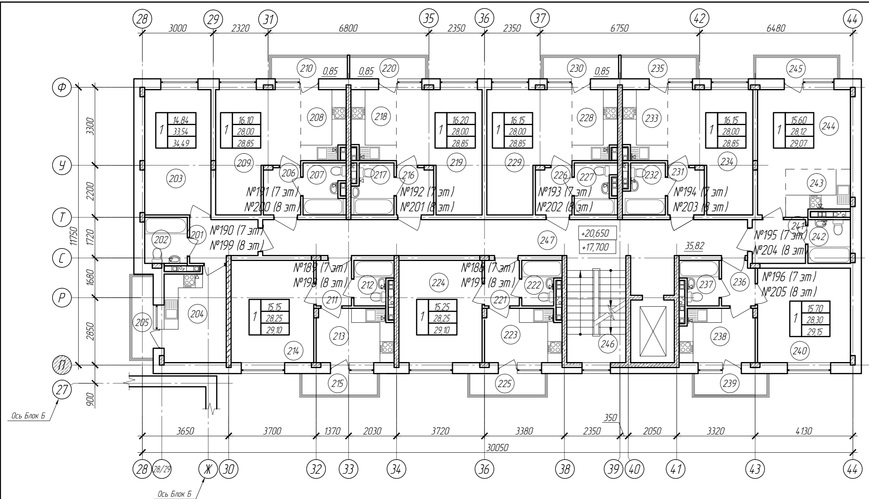
Компоновочная схема многоквартирного дома
